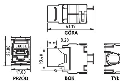
B. Profile modułu Keystone. Wymiary w mm
