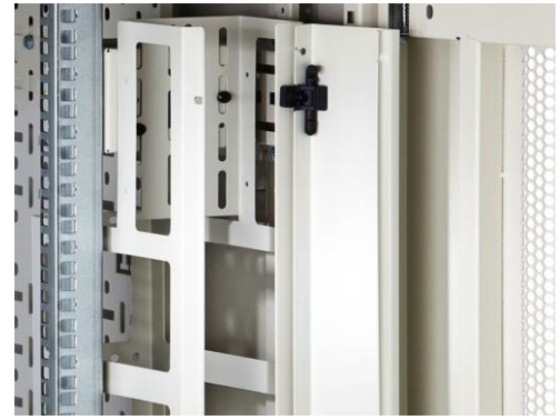
Uchwyty kablowe pionowe wysokiej gęstości
