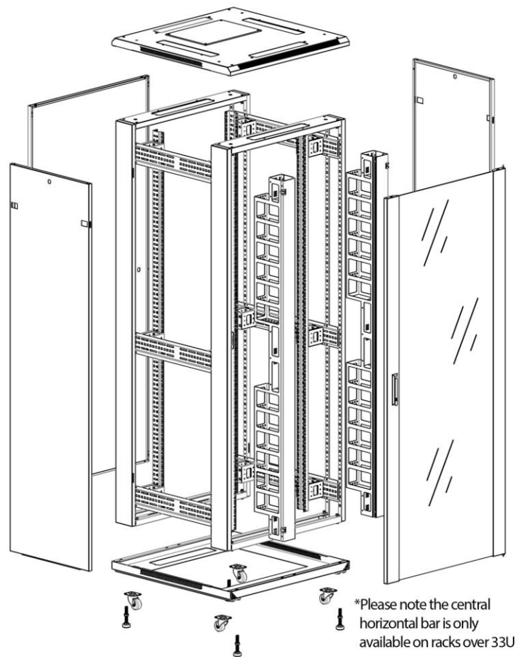
Zdemontowane osłony boczne na zatrzask
